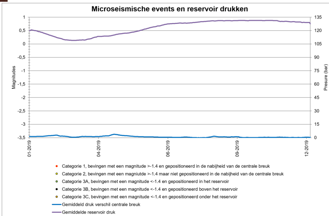
Figuur 2 Microseismische waarnemingen gedurende de rapportage periode van januari 2019 tot en met december 2019.
