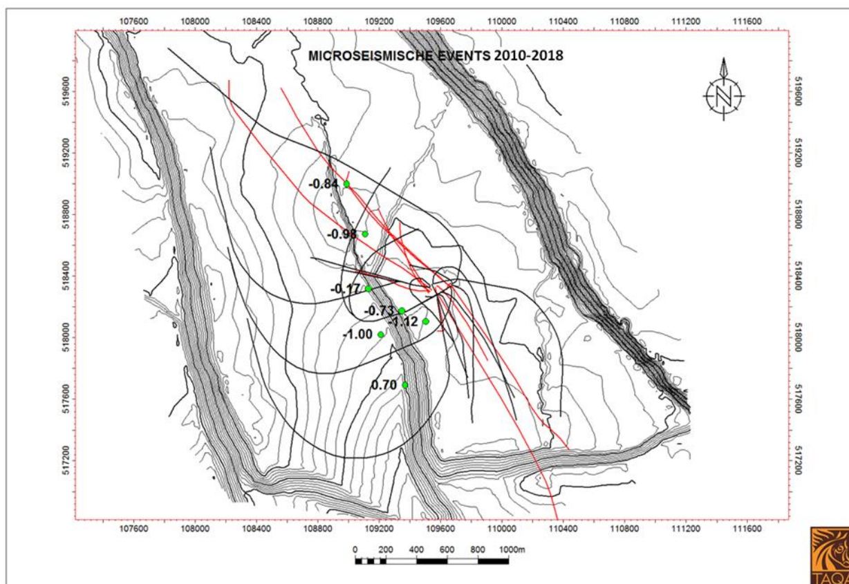
Figuur 1 Dieptekaart op Top Rotliggend niveau, met categorie-I trillingen ( M > -1,4 ) geprojecteerd In figuur 1 in zijn de locaties van de categorie 1 events aangegeven met groene rondjes. De magnitudes van de bevingen staan naast iedere locatie vermeld. De trajecten van de oude Bergermeer putten zijn in rood aangegeven en de trajecten van de nieuwe Bergermeer putten in zwart.
