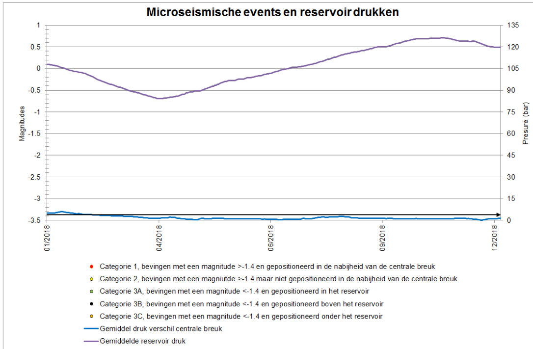
Figuur 2 Microseismische waarnemingen gedurende de rapportage periode van januari 2018 tot en met december 2018.
