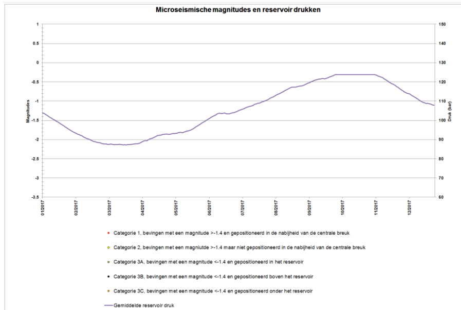
Figuur 2 Microseismische waarnemingen gedurende de rapportage periode van januari 2017 tot en met december 2017.
